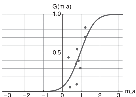
(a) H16 入学—H18 年新司 ( \beta = 1.86, T_A = 0.948 )
