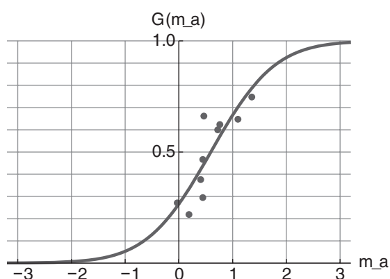
(d) H19 入学—H21 年新司 ( \beta = 1.32, T_A = 0.594 )
