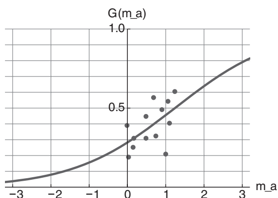
(b) H17 入学—H19 年新司 ( \beta = 0.48, T_A = 1.241 )
