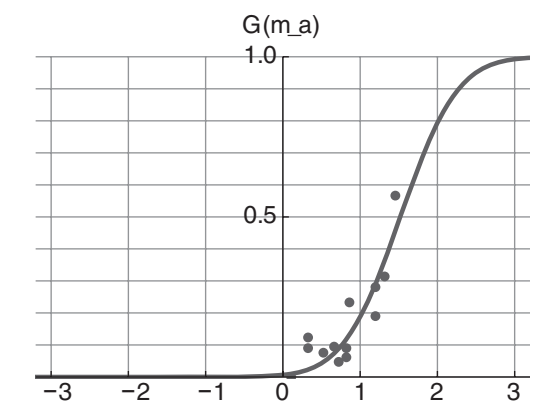
(e) H16 入学—H19 年新司 ( \beta = 2.25, T_A = 1.521 )
