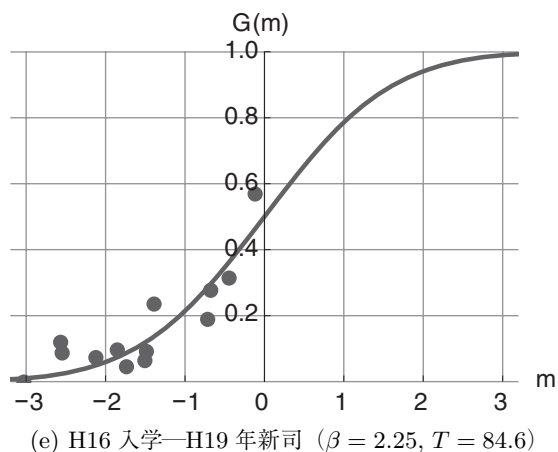
図 2 入学者の適性試験得点の平均点 m の大学院における新司法試験合格率 G(m) と実測値 ((a)~(d) は既修 (i)~(iv) のグラフ, (e) は未修 (v) のグラフを示す.)
